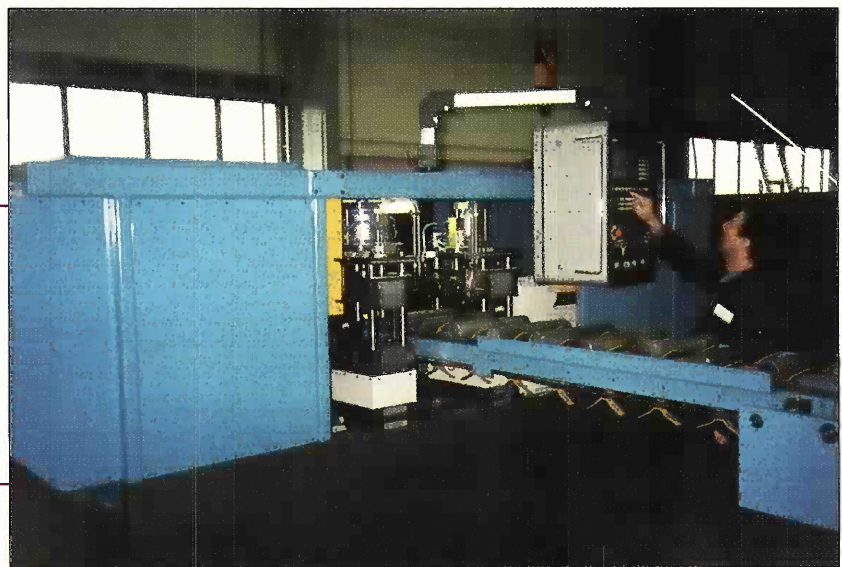
WIAP® DM2-A-H ZM » Abläng- und Andrehmaschine für Rohrbearbeitung, Bohrerfabrikation Taktzeit 22 sek, Lieferland Schweiz
