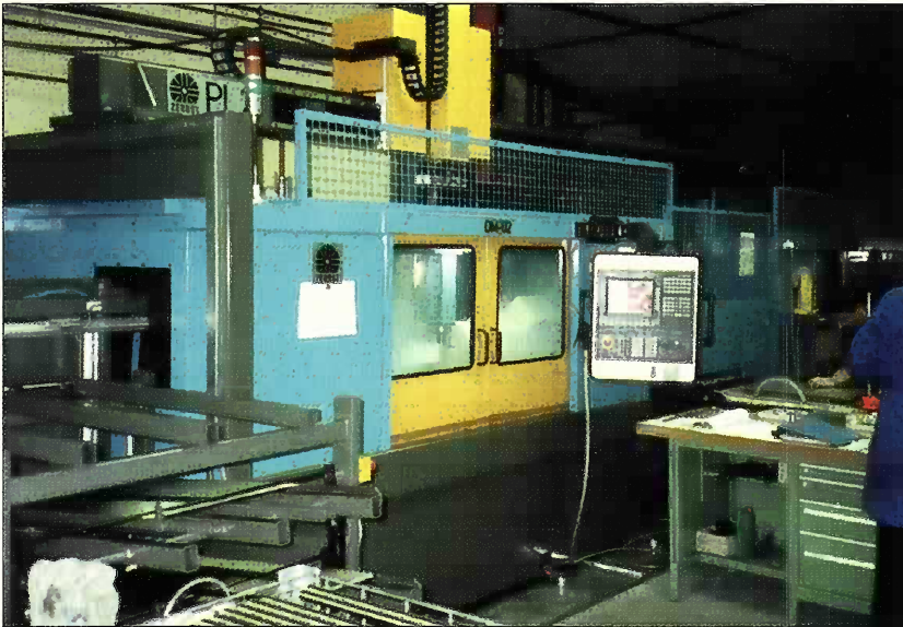
« WIAP® DM2-A-H Doppelseiten Drehmaschine eingesetzt für Fahrz. Industrie. Taktzeit 40 sek, Lieferland Deutschland
