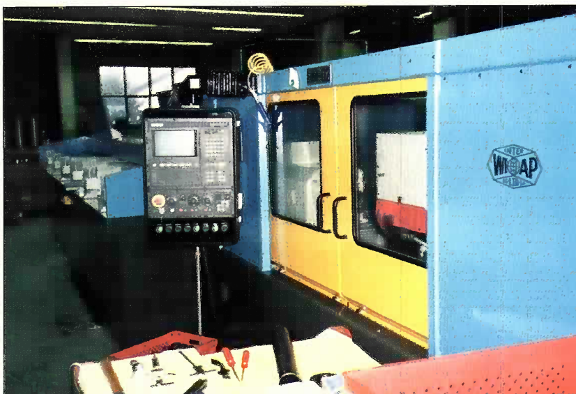
« WIAP® DM2-A-H HM Rohrbearbeitungsmaschine Rohrlänge 6 m für Bohrerhersteller Lieferland Schweiz
