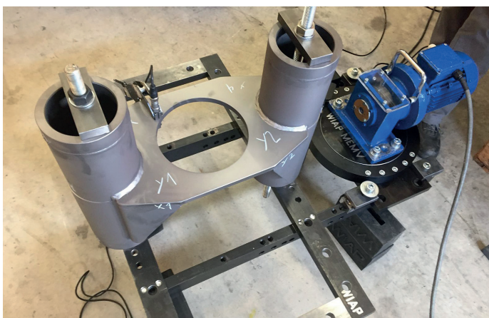
Eine Mehrfach-Aufspannvorrichtung, Kundenteil von Thommen Safenwil.
