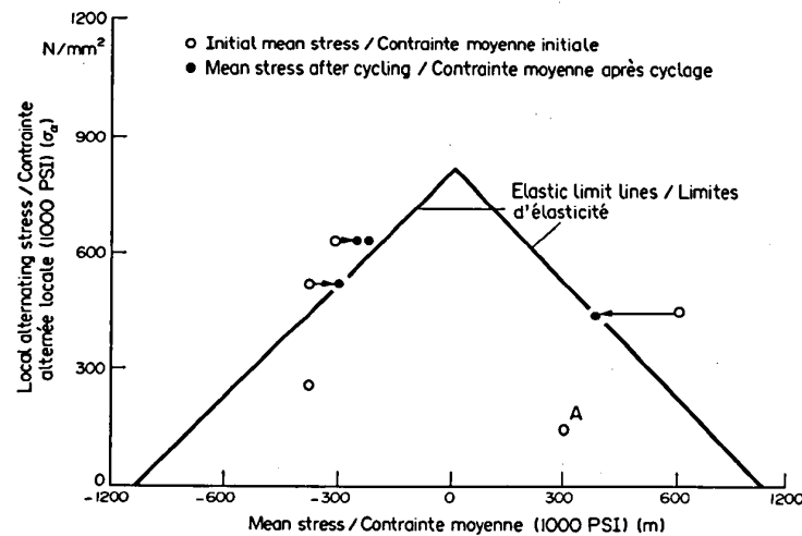
Fig. 1. Local alternating stress as a function of the mean stress/Contrainte alternée locale en fonction de la contrainte moyenne
