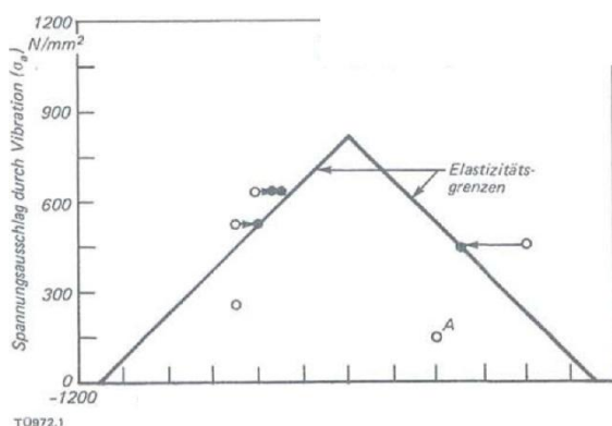
Bild 1: Zusammenhang zwischen verbleibender Eigenspannung und Höhe der Spannungsamplitude beim Vibrieren.
